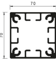
Staander
