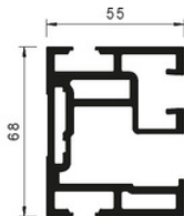
Geleiderrail
